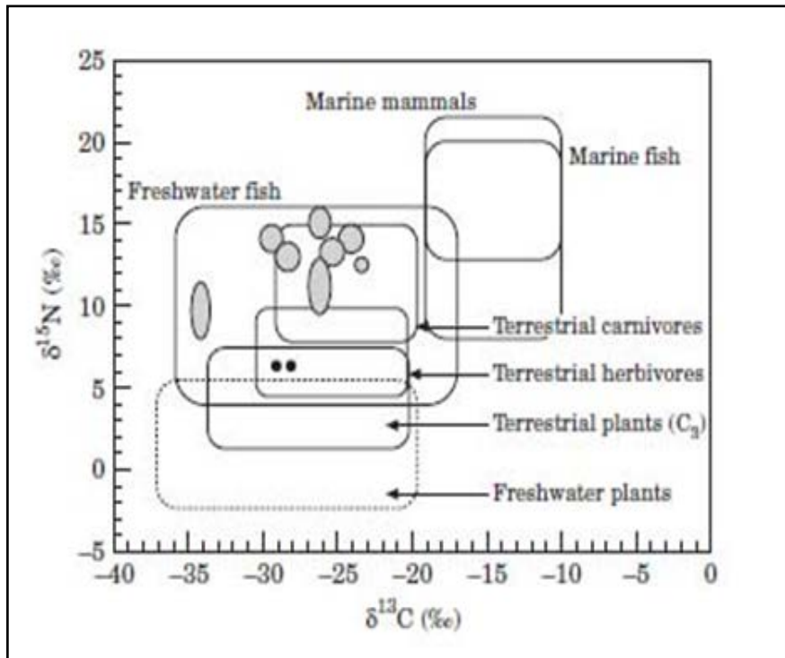
شکل ۳. تنوع‌های طبیعی ایزوتوپ 13C و δ و δ 15N در منابع اصلی رژیم غذایی در اوراسیا (جرح و تعدیل از: Bo-، 1997 cherens).
