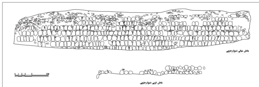
نقشه ۵. نمایی از دیوار جنوبی بنای تاریخی سرماج (ترسیم از م. احمدی، ۱۳۸۵). ◀
