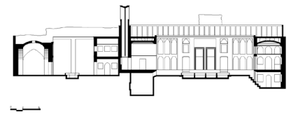
▲ نقشه ۲. مقطع الف-الف: خانه‌ی ملک‌زاده (آرشیو اداره‌ی کل میراث‌فرهنگی، صنایع‌دستی و گردشگری استان یزد، ۱۳۸۵).
