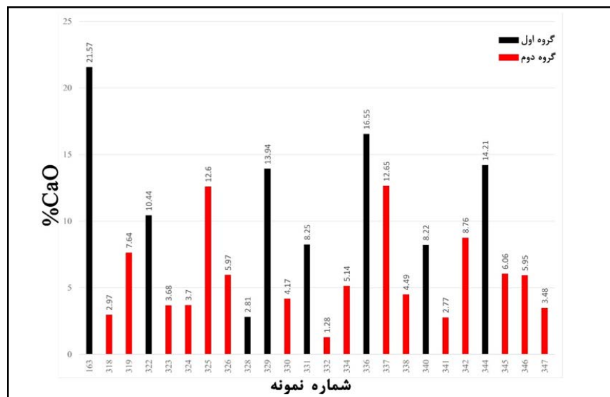
► شکل ۳. نمودار ستونی میزان CaO در ترکیب نمونه‌های دو گروه سفال‌های محوطه‌ی ده‌دومن (نگارندگان، ۱۳۹۷).
