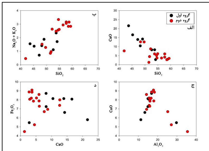
شکل ۴. الف) نمودار پراکندگی \text{SiO}_2 در برابر \text{CaO} ، ب) \text{SiO}_2 در برابر \text{Na}_2\text{O} + \text{K}_2\text{O} ، ج) \text{Al}_2\text{O}_3 در برابر \text{CaO} ، د) \text{CaO} در برابر \text{Fe}_2\text{O}_3 براساس نتایج آنالیز XRF نمونه‌های سفالی محوطه‌ی ده‌دومن (نگارندگان، ۱۳۹۷). ◀
