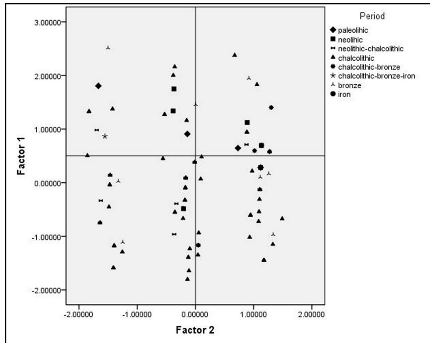
► نمودار ۱. ماتریس همبستگی عامل‌های یک (محیطی) و دو (ارتباطی) مورد مطالعه (عسکری‌پور، ۱۳۹۸).
