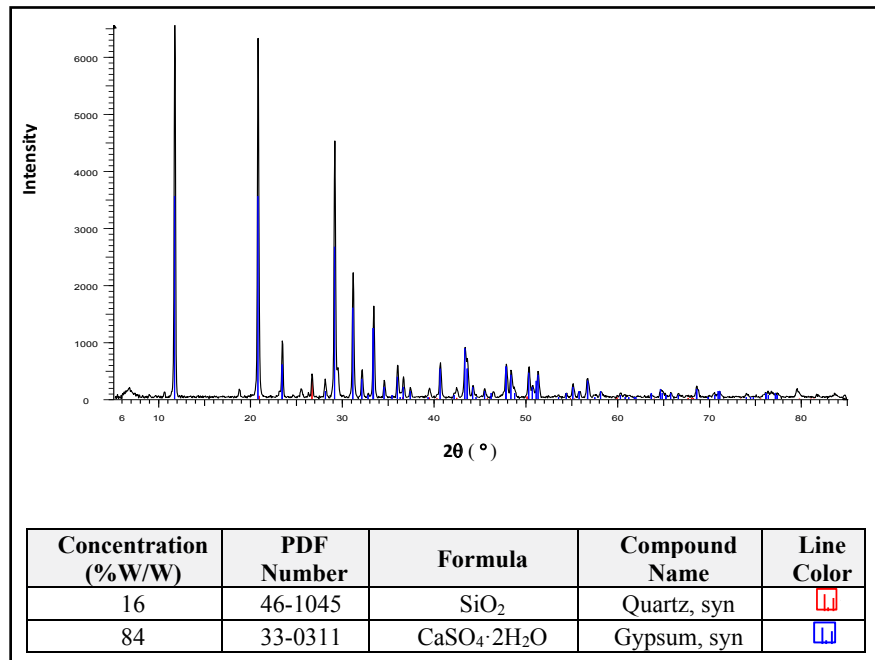
► شکل ۸. طیف پراش پرتو ایکس (XRD) ملات گچ‌بری راهروی طبقه اول (نگارندگان، ۱۳۹۹).
