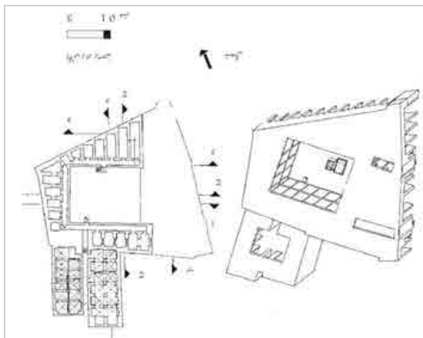
► شکل‌های ۶ و ۷. پرسپکتیو و نقشه‌ی طبقه‌ی زیرزمین کاروانسرای حاج صفرخانی همدان (زارعی، ۱۳۷۶: ۲۳۱).
